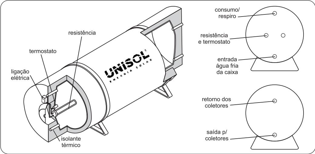
Reservatório térmico de aço inoxidável
