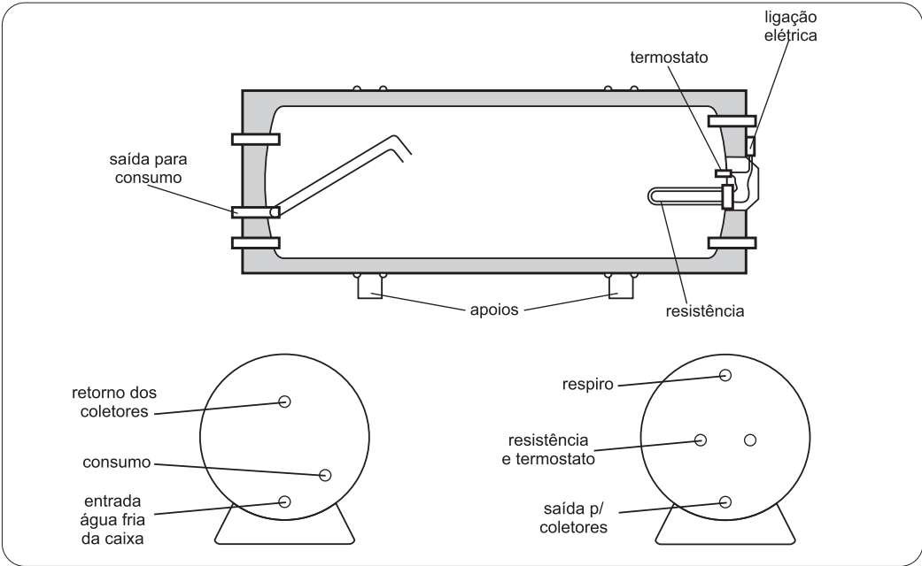
Reservatório térmico de aço inoxidável (A.I.) Nível
