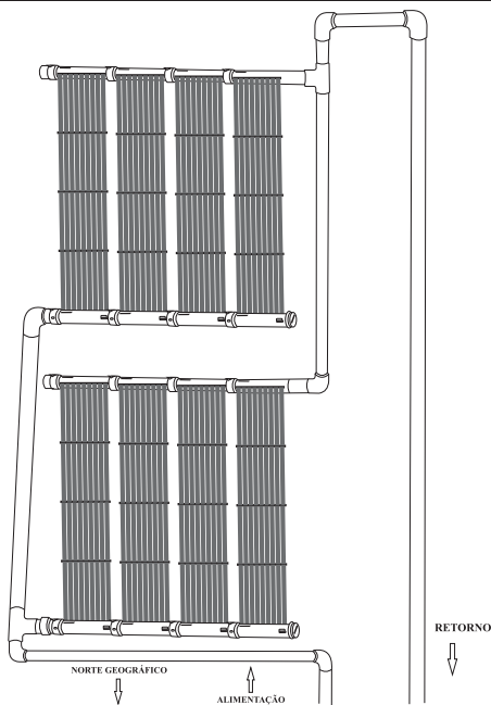
Ligação em paralelo
