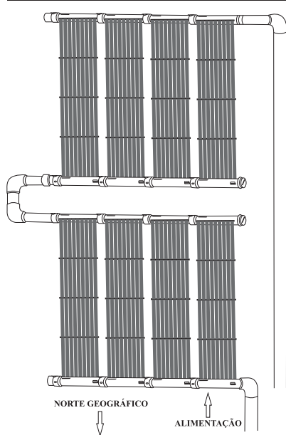
Ligação em série
